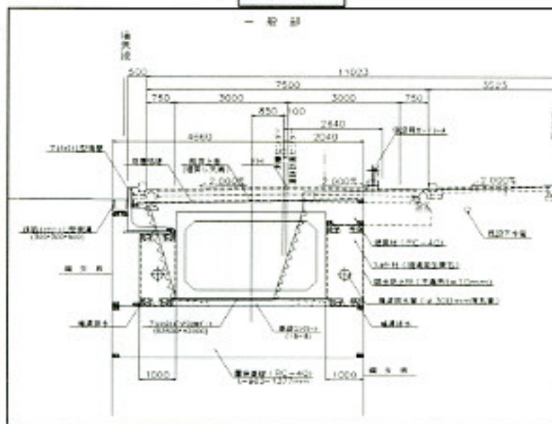
標準断面図
