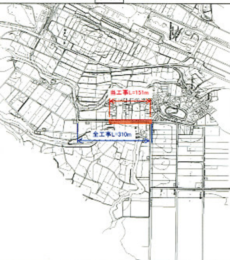
平面図
